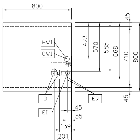
Boven aanzicht
